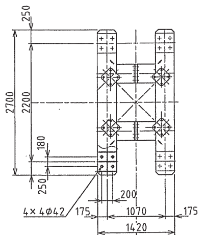
A 矢視 (S=1/50)
