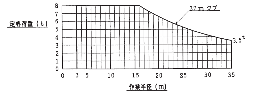
性能線図
