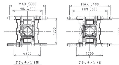
台座平面図
