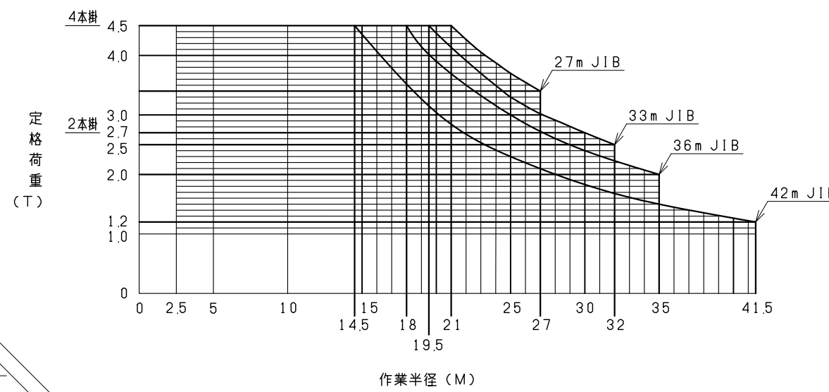
性能曲線
