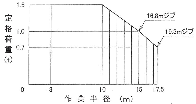
定格荷重線図
