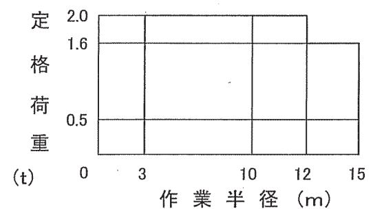
定格荷重線図 17.0mジブ
