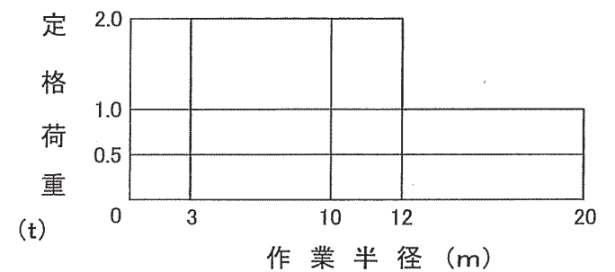
定格荷重線図 17.0mジブ
