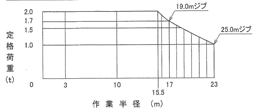
定格荷重線図
